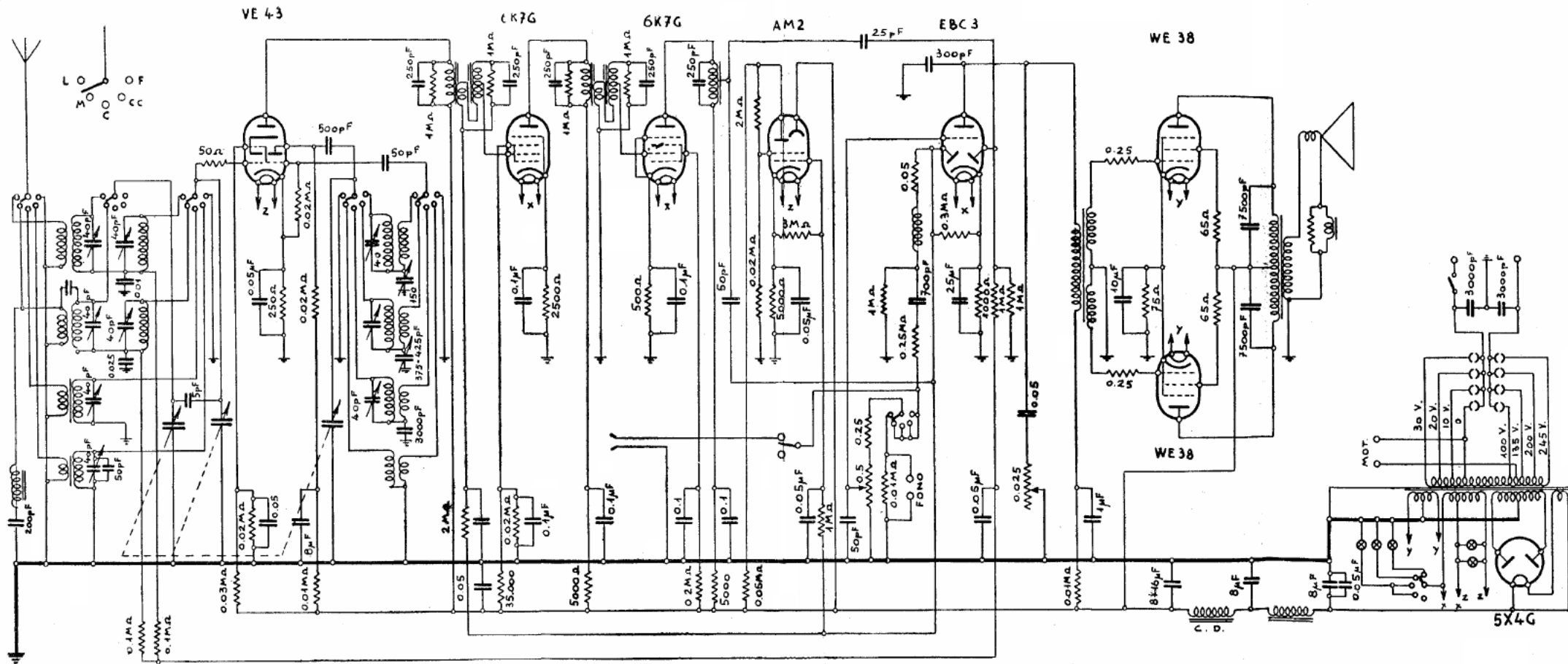
LA VOCE DEL PADRONE. — Mod. « Marcon 1756 ». Telaio Voce del Padrone mod. 561. — Produzione 1899-1940. — Media frequenza: 485 kHz. — (Questo ricevitore è descritto in Moderna Supereterodina, 5ª ediz.) Il mod. « 1756 A » corrisponde al mod. « 1756 » con la differenza che al posto del condensatore fisso di 700 pF nel circuito del diodo rivelatore della EBC 3 sono stati messi due condensatori in serie, uno da 3000 pF e l'altro di 350 pF, quest'ultimo può venir cortocircuitato dando luogo al comando « Fedeltà ».
